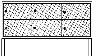
14. ábra 6 nyúl elhelyezésére alkalmas ketrec vázzata
